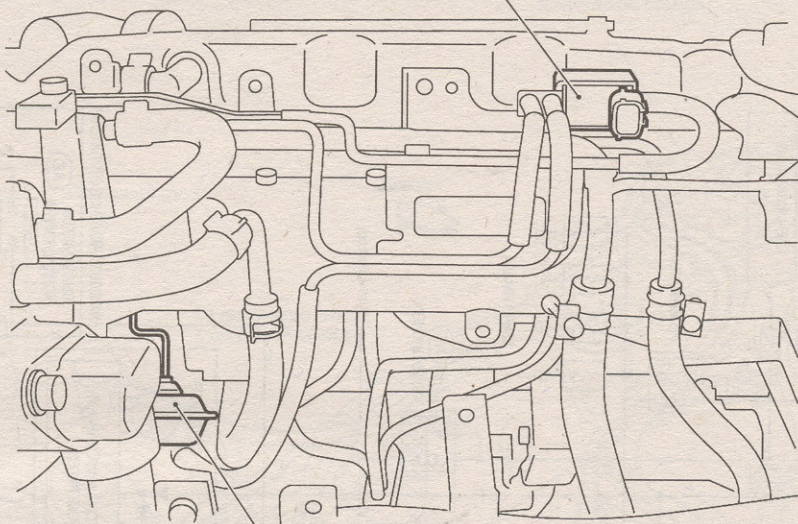
Вакуумный исполнительный элемент клапана завихрения
