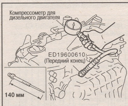
⊗: 18 - 21 Nm (1,8 - 2,2 кг-м)
