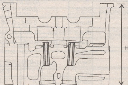
Номинальная высота головки цилиндров: H = 153,9 - 154,1 мм
